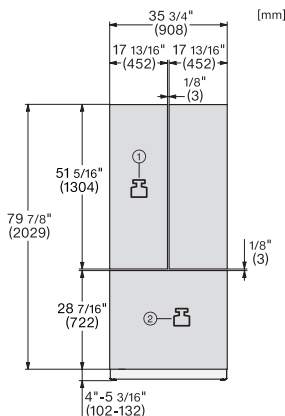
KFMC3642FD, KFMC3844FD, MasterCool III, Ansicht von vorne (*Fußnote) (Skizze)
