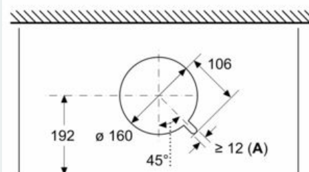
Maße in mm Ansicht von oben
