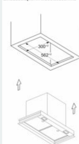
Maße in mm Einbaubeispiel in Möbelausschnitt
