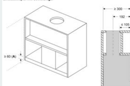
Maße in mm Einbaubeispiel mit Gewürzregal
