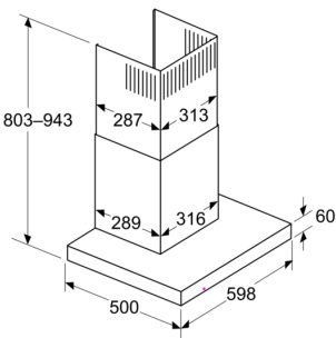
Maße in mm Ansicht Umluft
