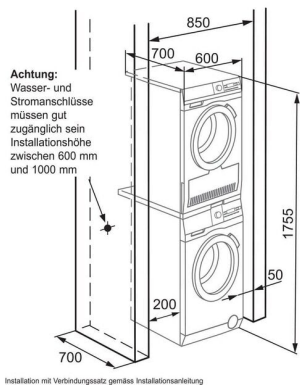
Belüftungsbeispiel für Wasch-Trockensäule Nischeneinbau ohne Tür
