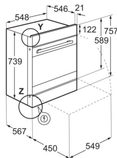
Einbaubackofen/Einbaubernd EB7.../EH7...
