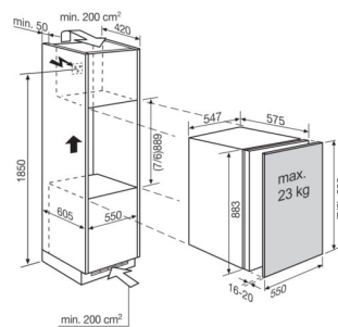
IK159S Möbelfront auf Gerätetür verschraubt
