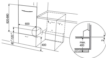
GA60SLVC/SLVS/GLVC/GLVS/GLV/LV/KV - eingebaut in Hochschrank mit Gleitürmontage
